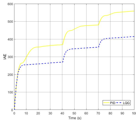
(b) IAE profile.
